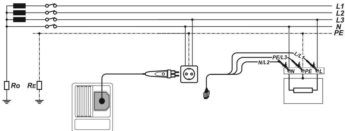
Aansluiting van de als optie verkrijgbare Commander meetstekker (044149) en de 3-aderige meetkabel
