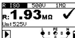
Afbeelding 5.7: Voorbeeld isolatieweerstandsmeting
