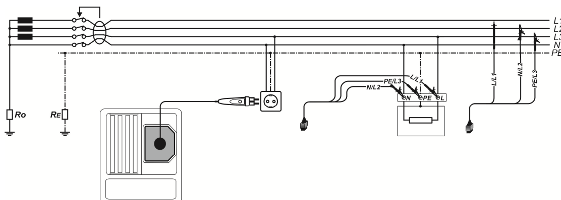
Afbeelding 5.3: Aansluiting van de optionele Commander-teststekker (044149) en de 3-geleider testdraad in het een-/driefasesysteem
