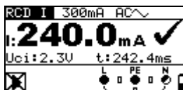
Afbeelding 5.20: Voorbeeld activeringsstroommeting
