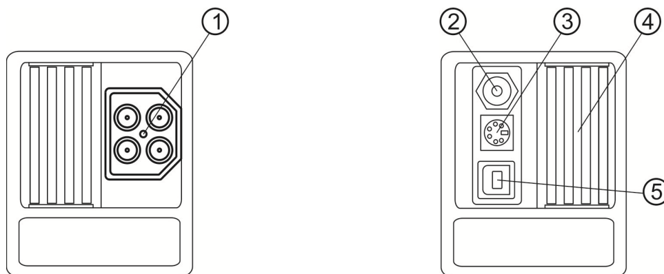
Afbeelding 3.2: Aansluitpaneel
