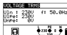
Afbeelding 5.1: Spanning in eenfasesysteem
