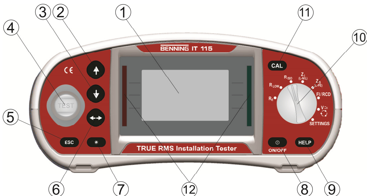
Afbeelding 3.1: Voorzijde
