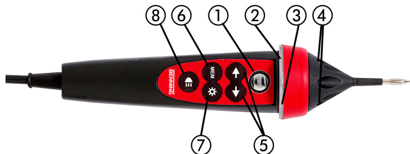
Afbeelding C.1: Voorzijde van Commander-testpen, schakelbaar met TEST-toets (044155)
