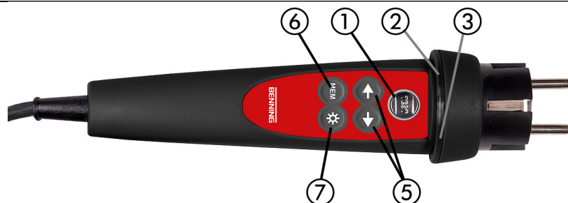
Afbeelding C.2: Voorzijde van Commander-teststekker voor stopcontact met randaarde (schakelbaar met TEST-toets) (044149)
