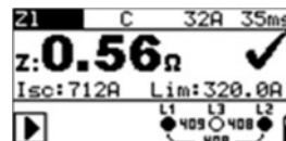
Afbeelding 5.29: Voorbeeld leidingsimpedantiemeting
