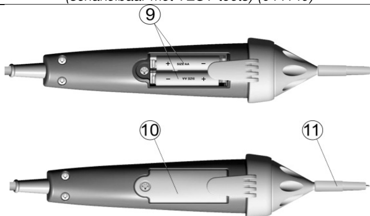
Afbeelding C.3: Achterzijde van Commander-testpen, schakelbaar met TEST-toets (044155)
