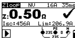
Afbeelding 5.25: Voorbeeld lusweerstandsmeting
