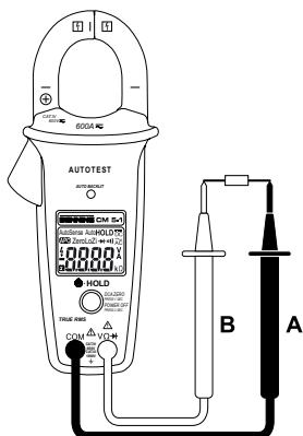
Bild 4: Widerstandsmessung Fig. 4: Resistance measurement Fig. 4: Mesure de la résistance Fig. 4: Medición de resistencia Obr. 4: Měření odporu Σχήμα 4: Μέτρηση αντίστασης 4. ábra: Ellenállásmérés III. 4: Misura di resistenza Fig. 4: Weerstandsmeting Rys. 4: Pomiar rezystancji Imaginea 4: Măsurarea rezistenței Рис. 4: Измерение сопротивления Fig. 4: Resistansmätning Resim 4: Direnç ölçümü
